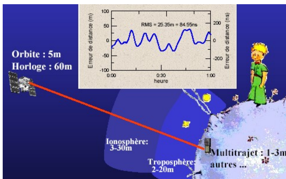
Illustration 5 : Les erreurs du GPS
