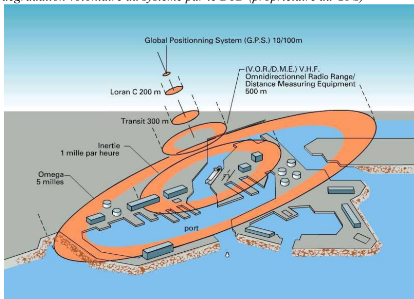
Illustration 11 : Précision des différents systèmes de radiopositionnement
