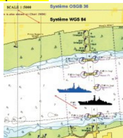
Illustration 12 : Écart de position entre le WGS 84 et l'OSGB 86
