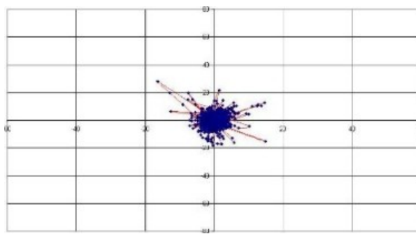
Illustration 10 : Variation d'un point fixe dans le temps vu par un GPS différentiel
